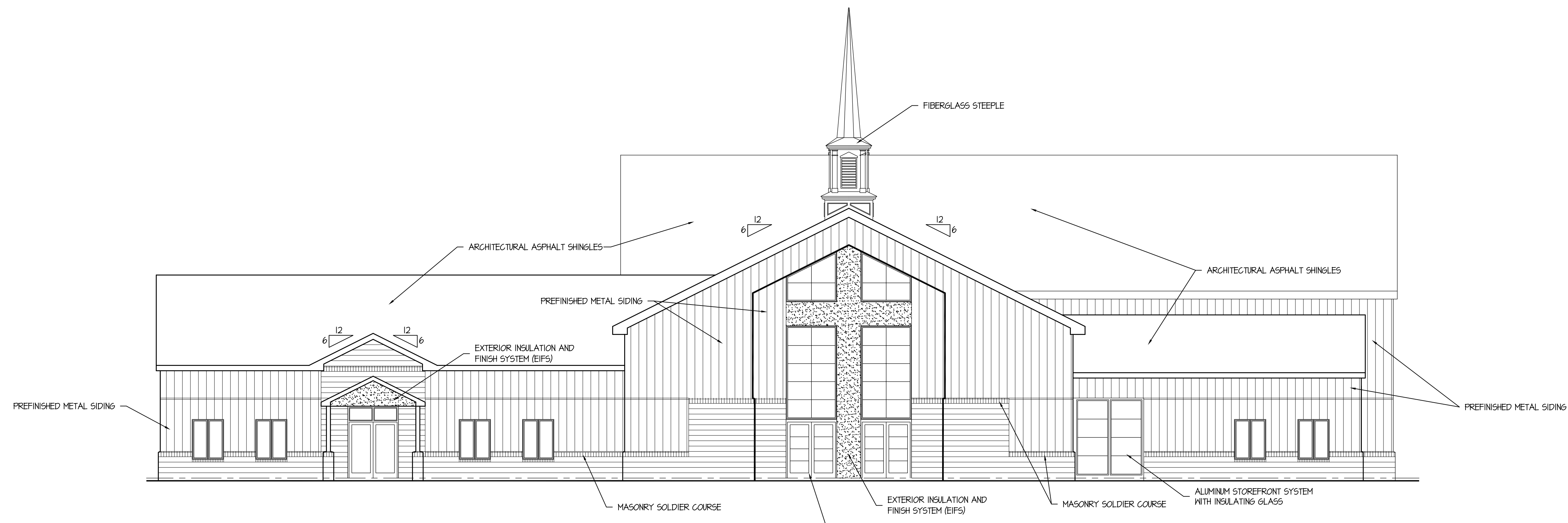
FRONT EXTERIOR ELEVATION SCALE: 1/8" = 1'-0"
